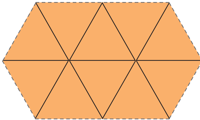
Triángulos equiláteros
